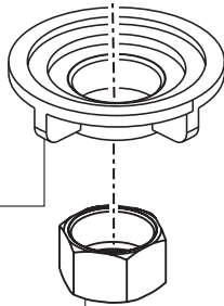
RP5861 Coupling Nuts (Optional, not included) Tuercas de Acoplamiento (Opcional, no incluido) Écrous de Raccordement (Option, non inclus)
